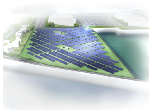
白石ソーラーウェイ完成予想図
